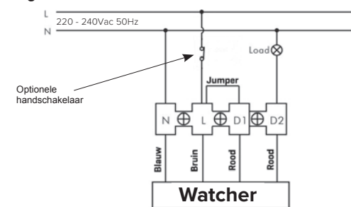
Fig. 3: Aansluitschema A
