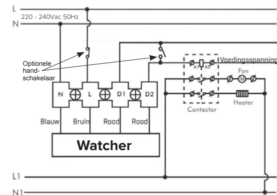
Fig. 3: Aansluitschema B
